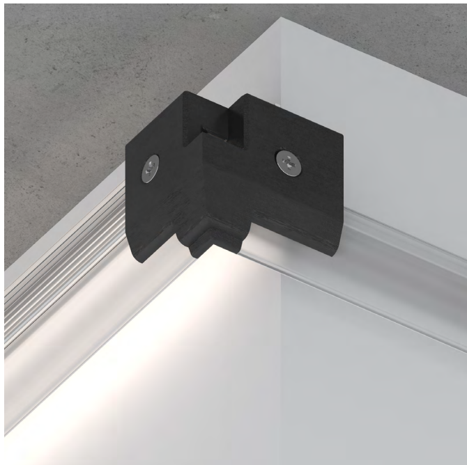
Парящий-теновой, внешний угол, левый
